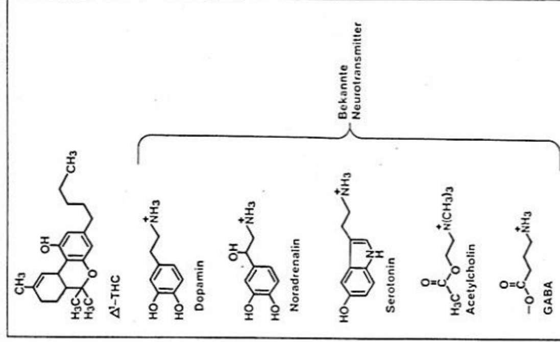
Darstellung 4: Vergleich von \Delta^1 -Tetrahydrocannabinol mit den Strukturen bekannter Neurotransmitter
