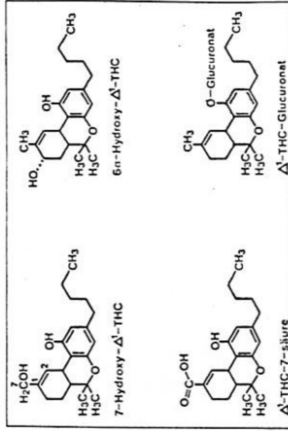
Darstellung 6: Strukturen wichtiger Metabolite von \Delta^1 -THC
